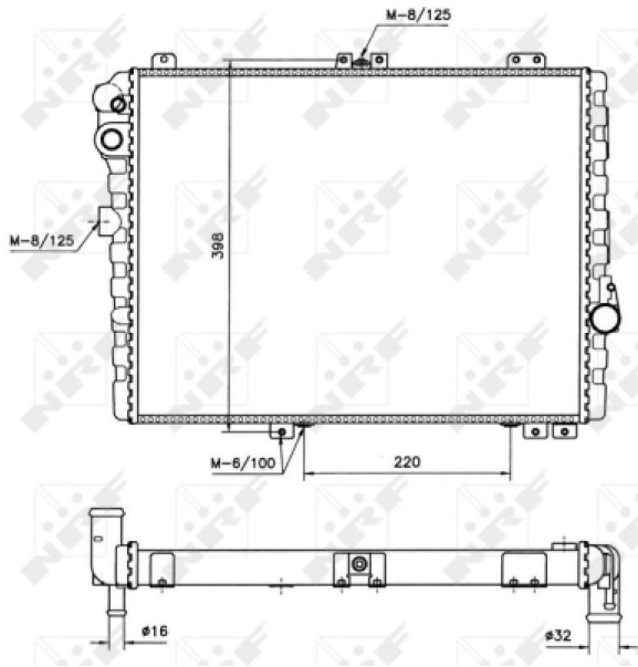
Motor radiator Audi 90 5 cil
